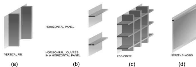
Slika 6. Osnovni tipi vertikalnih (a), horizontalnih (b), kombiniranih (c) ter ploskovnih senčil (d) (povzeto po [Žegarac Leskovar, 2013]).
