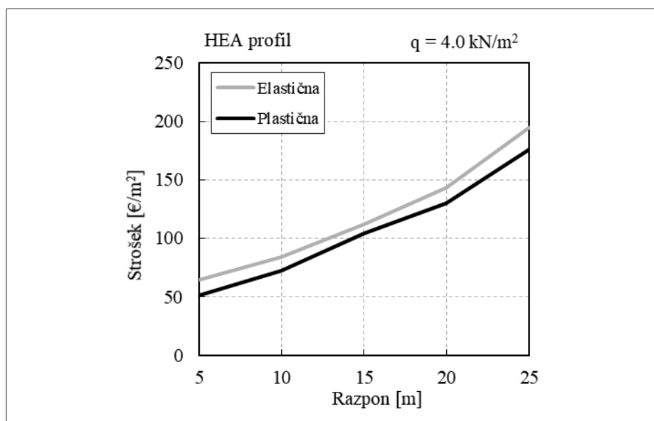
Slika 10 • Diagram lastnih izdelavnih stroškov sovprežnega stropnega sistema z jeklenimi HEA-profilom pri plastični in elastični odpornosti prereza.
