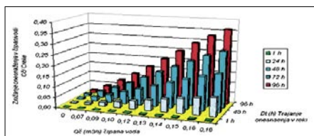
Slika 8 • Redukcija in naraščanje inertnega onesnaženja obrežnega filtrata v L = 100 m dolgi drenaži od črpane vode Q (m³/s) pri odmikih drenaže od brežine reke L1 = 75 m in L2 = 150 m pri trajanju onesnaženja od 0 do 96 ur
