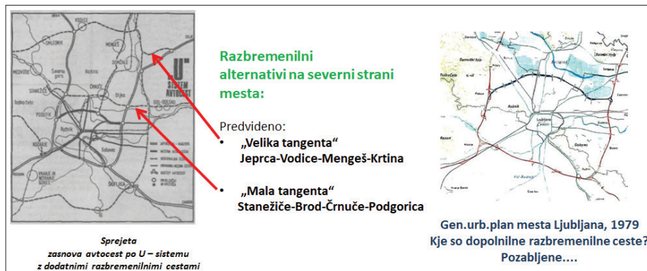
Slika 7 • Izbrani U-sistem AC okoli LJ – Generalni urbanistični plan LJ 1979 (Vira: (Gaberšček, 1978) in (DRC, 2014)).
