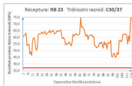
Slika 25: Rezultati preizkusov tlačnih trdnosti betona C30/37, XC4, XD3, Dmax 32, S4, PV-II.
