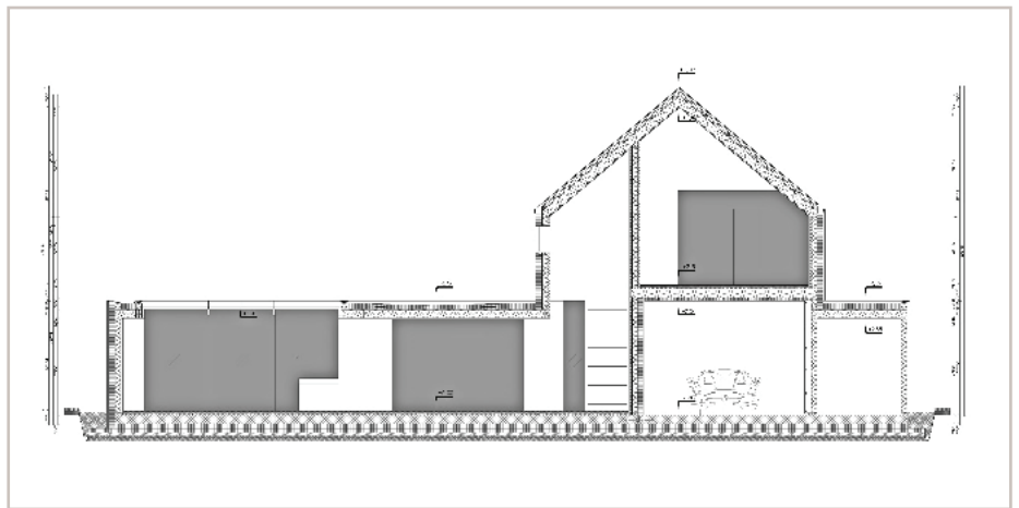
Slika 8 Vzdolžni prerez.
