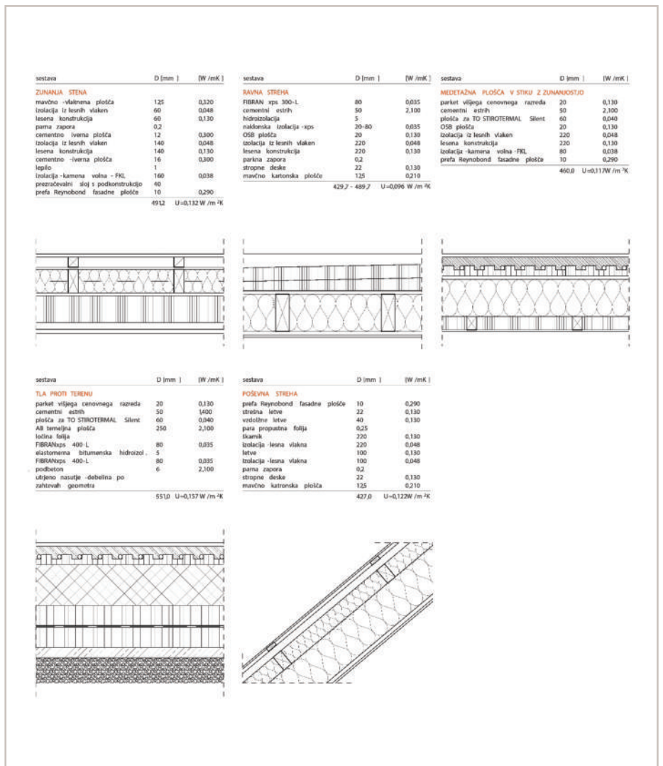
Slika 9 Sestave elementov termičnega ovoja.
