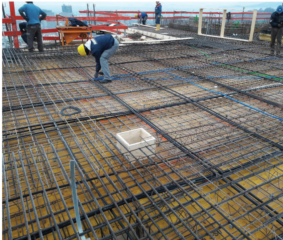
Slika 14: Polaganje armature in kablov za prednapenjanje ter zaščitnih cevi inštalacij pred betoniranjem plošče.
