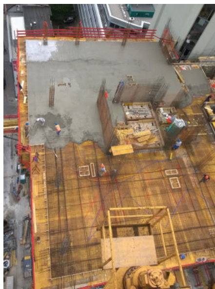
Slika 16: Betoniranje AB-plošče, pogled z žerjava.
