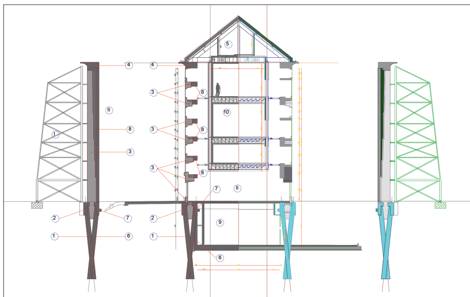
Slika 6 • Karakteristični prerez z rekonstrukcijskimi posegi.
