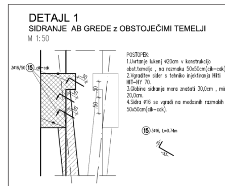
Slika 8 • Detajl AB-grede na zunanji strani temeljnega zidu.
