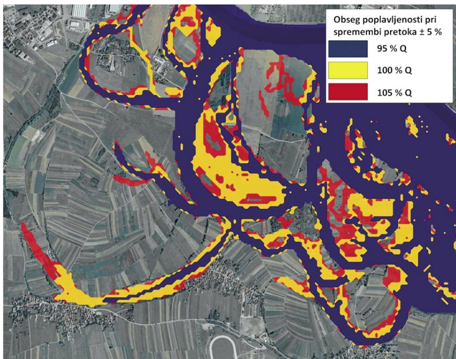
Slika 14 • Analiza vpliva računske negotovosti prikaže, koliko se spremeni obseg poplavljenosti, če spreminjamo računski pretok v mejah Q_{\text{RAČUN}} \pm 5\% (prelivanje Save na desno poplavno območje)
