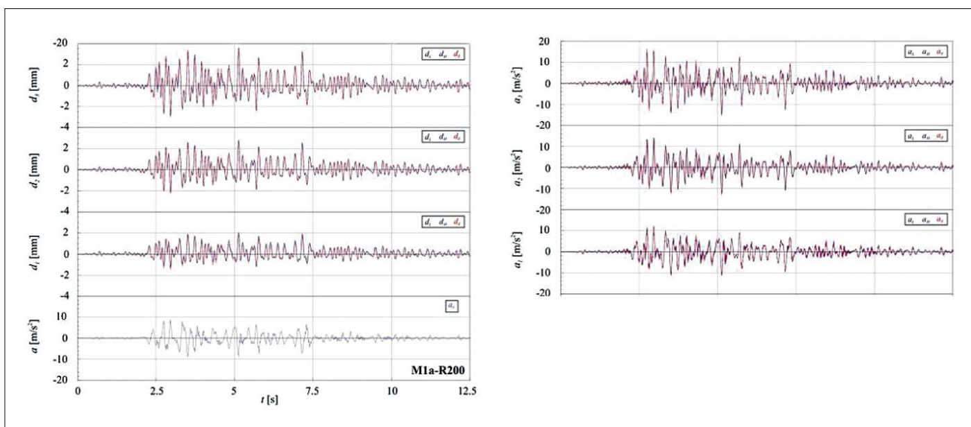
Slika 16 • Časovni potek odziva pomikov in pospeškov modela M1a med fazo preiskave R200
