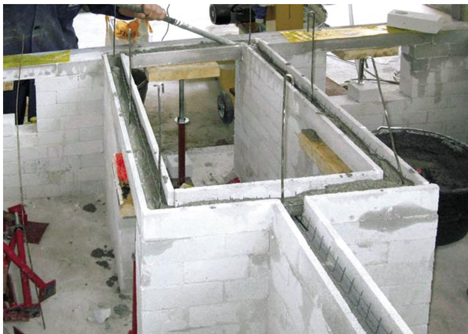
Slika 8 • Beli strop: betoniranje vodoravnih zidnih vezi in preklad
