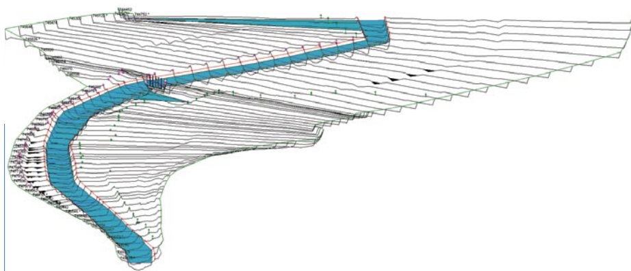
Slika 3 • Primer hidravličnega 1D-modela, ki z razširitvijo prečnih prereзов poenostavljeno zajame tudi poplavne površine (programska oprema HEC-RAS; FGG-KMTe)
