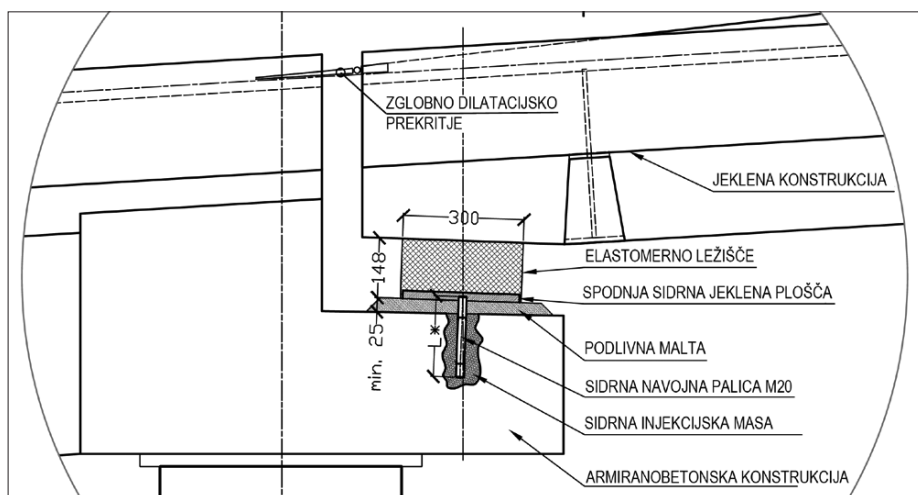
Slika 9 • Detajl prehoda prekladne konstrukcije nad vmesno podporo.
