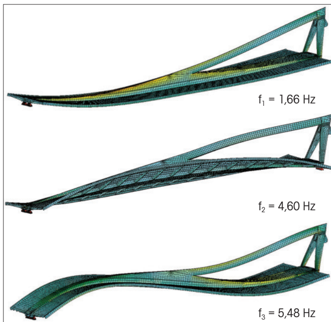
Slika 6 • Osnovne nihajne oblike konstrukcije.
