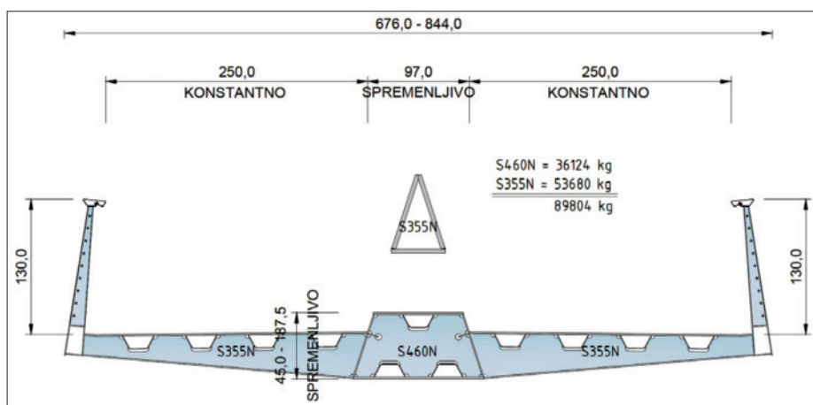
Slika 8 • Prečni prerez PZI.
